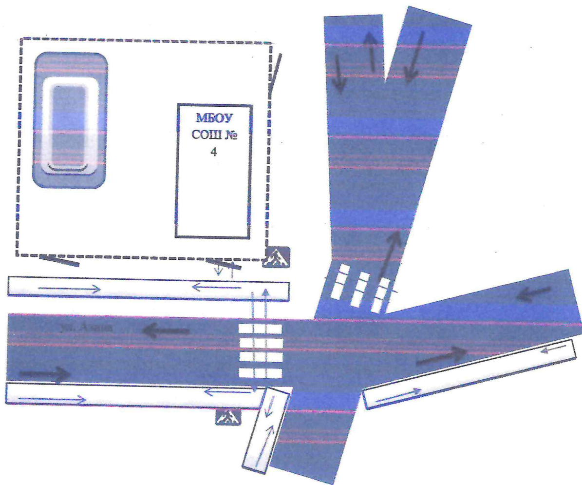
Схема организации дорожного движения в непосредственной близости от МБОУ СОШ № 4 с размещением соответствующих технических средств, маршруты движения детей.
